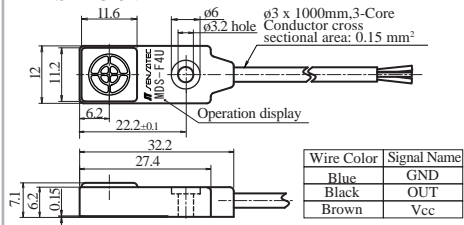
MDS-F4U-5V
