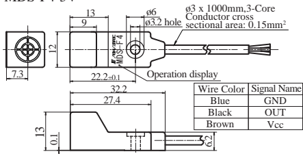
MDS-F4-5V
