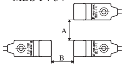
MDS-F4-5V
